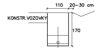
PŘ 1,2,3 (PŘÍČNÝ ŘEZ ULOŽENÍ ŘADU V SIL. III/2904): M 1 : 100
