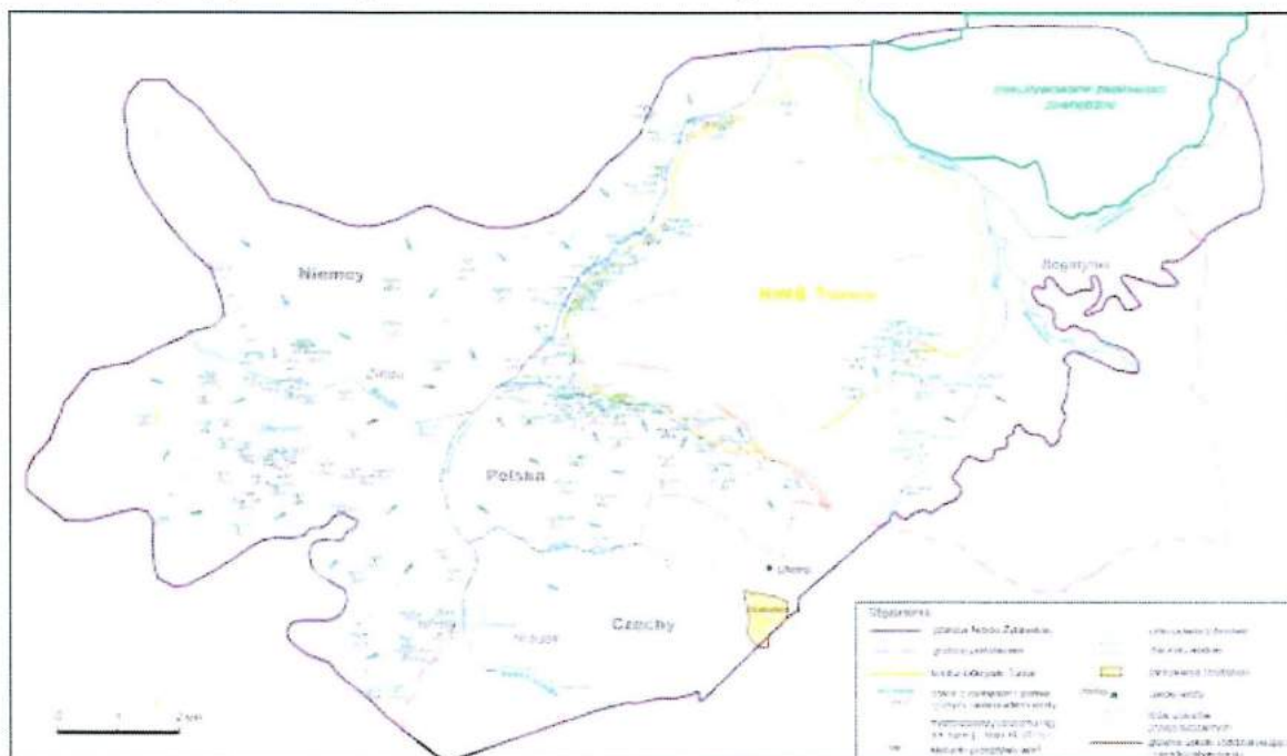
Obrázek č. 5 Mapa výšky vodní hladiny vodonosného útvaru hlušina – horní Ng – stav v IX/2015
