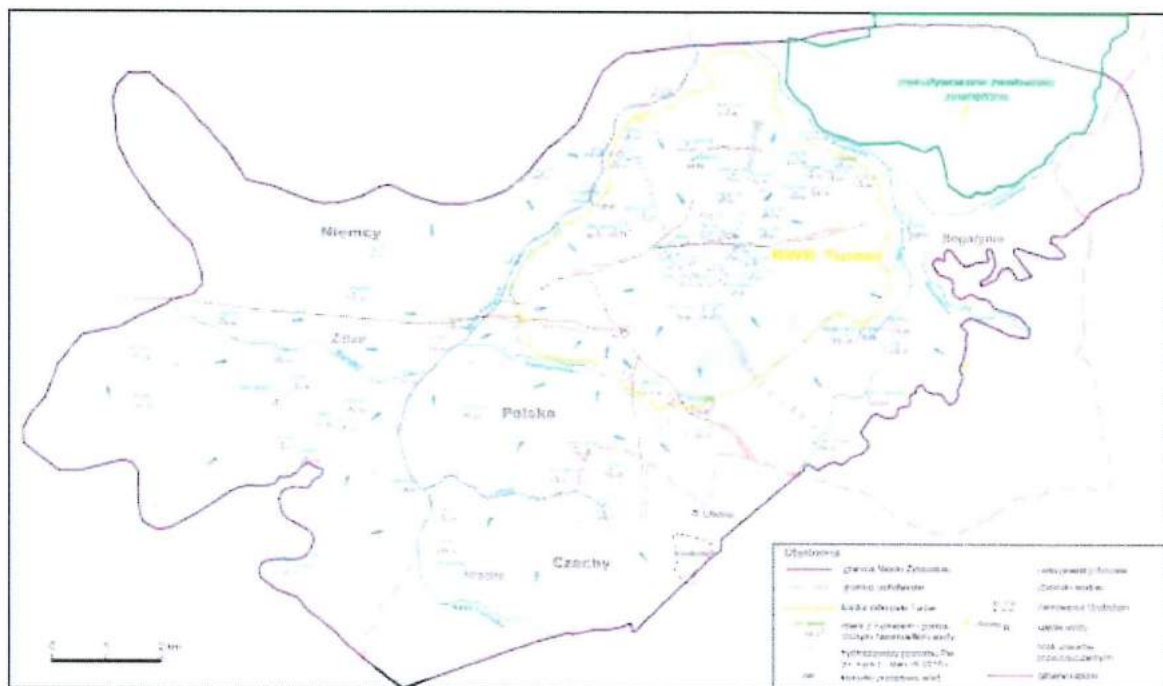
Obrázek č. 8 Mapa výšky vodní hladiny poduhelného vodonosného útvaru Pw – stav v IX/2015
