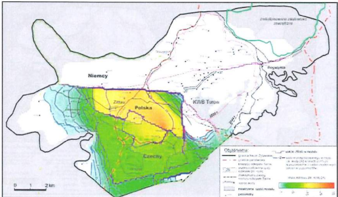
Obrázek č. 19 Mapa vzestupu vodní hladiny podzemní vody na úrovni Pw (vrstva č. 5) v letech 2015–2020 v důsledku funkce protifiltrační clony
