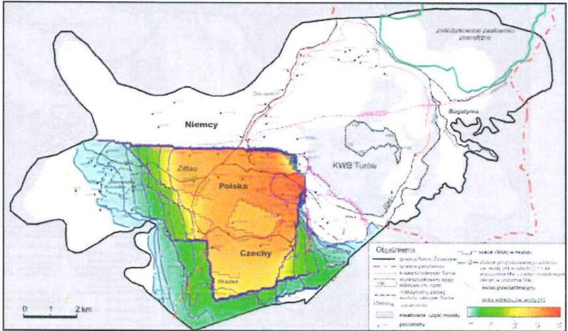
Obrázek č. 23 Mapa vzestupu vodní hladiny podzemní vody na úrovni Mw (vrstva č. 4) v letech 2015–2020 v důsledku funkce protifiltrační clony
