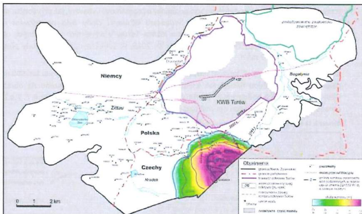
Obrázek č. 13 Vzestup vodní hladiny v oblasti jímání Uhelná (odběr Q=593 \text{ m}^3/\text{d} ) v mokřém období
