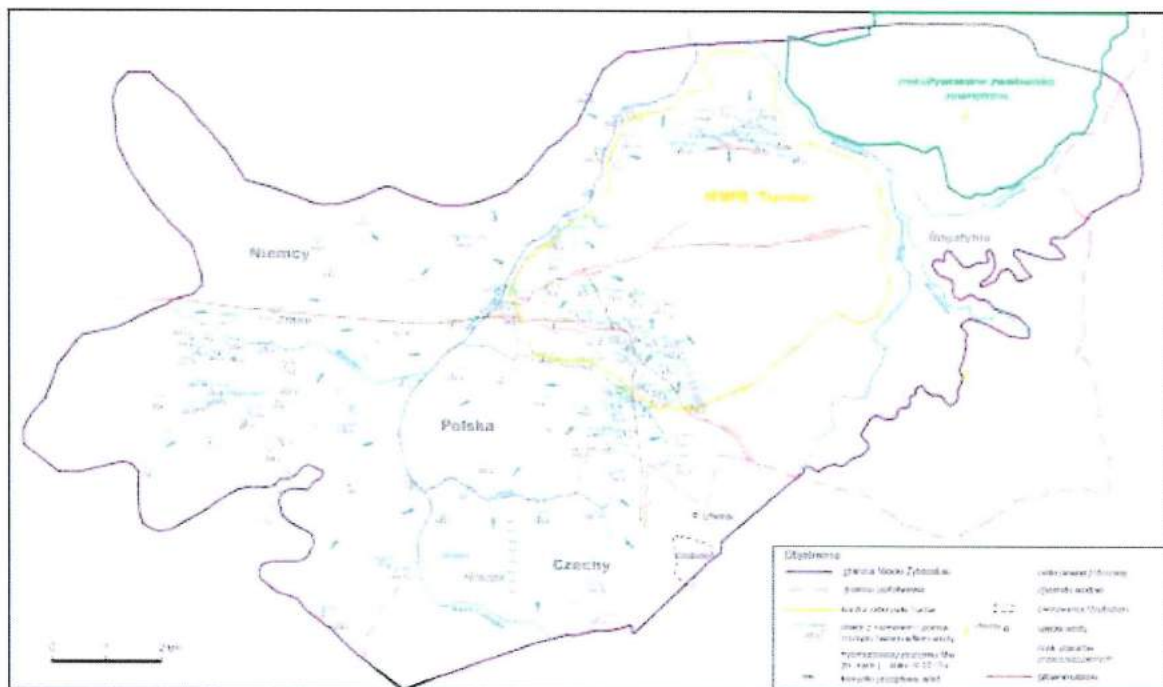
Obrázek č. 7 Mapa výšky vodní hladiny meziuhelného vodonosného útvaru Mw – stav v IX/2015
