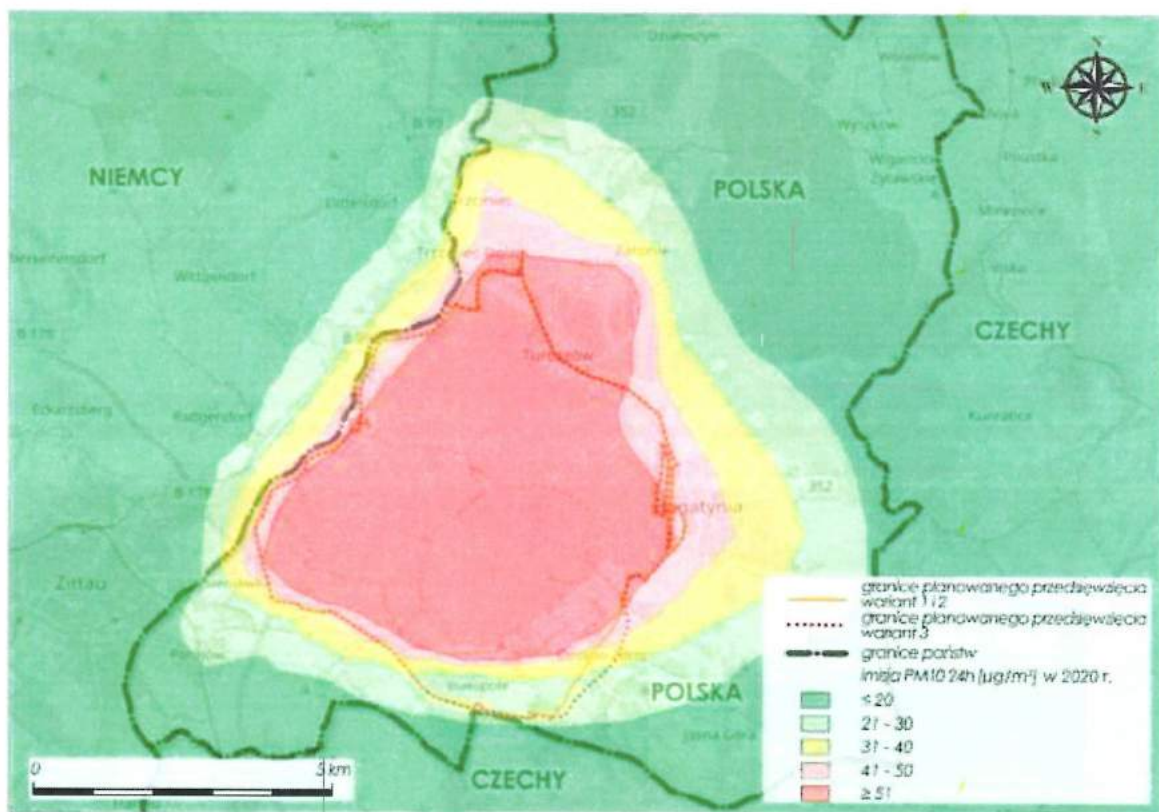
Obrázek č. 25 Rozložení imisí poléťavého prachu PM10 24h (max. 36) pocházejících z kumulovaných emisí v roce 2020
