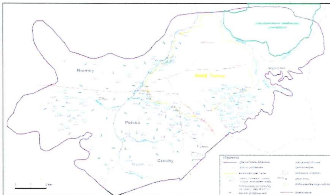
Obrázek č. 6 Mapa výšky vodní hladiny vodonosného útvaru hlušina – dolní Nd – stav v IX/2015
