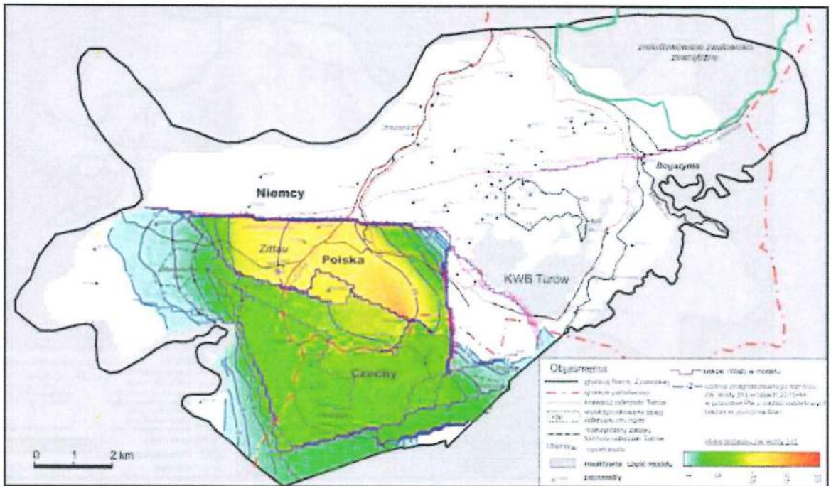
Obrázek č. 24 Mapa vzestupu vodní hladiny podzemní vody na úrovni Pw (vrstva č. 5) v letech 2015–2044 v důsledku funkce protifiltrační clony
